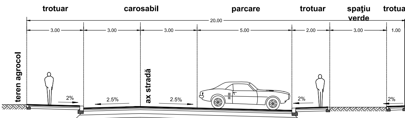
Secțiunea 8 Profil transversal
