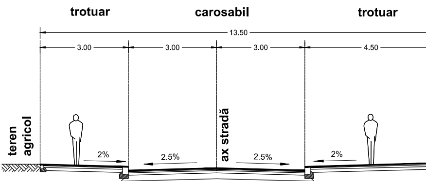
Secțiunea 6 Profil transversal
