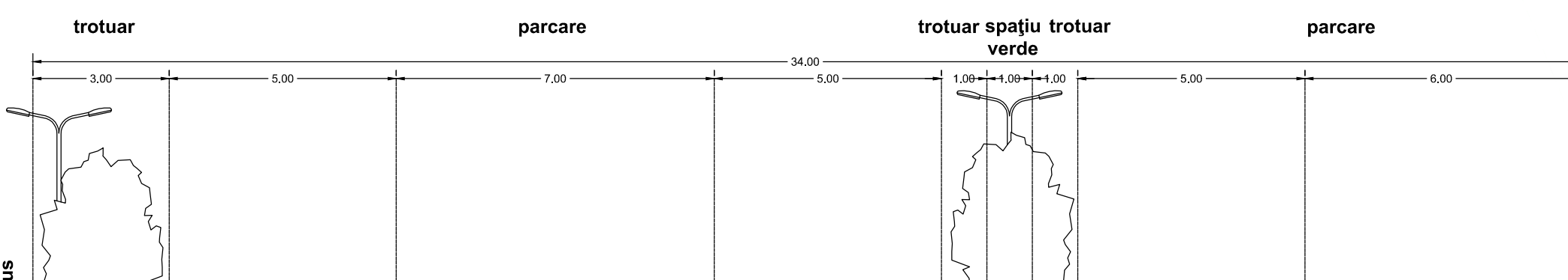
Secțiunea 8 Profil transversal
