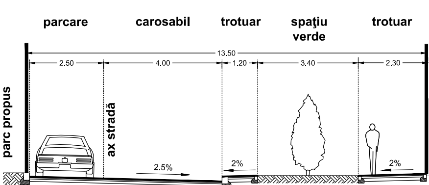
Secțiunea 4 Profil transversal
