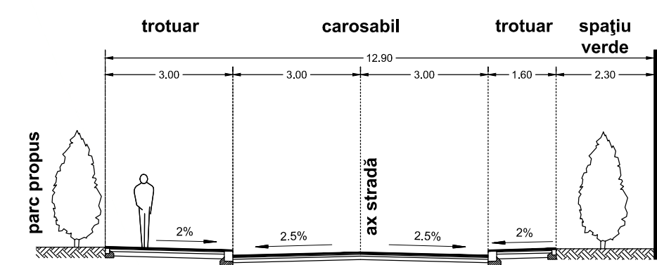
Secțiunea 3 Profil transversal
