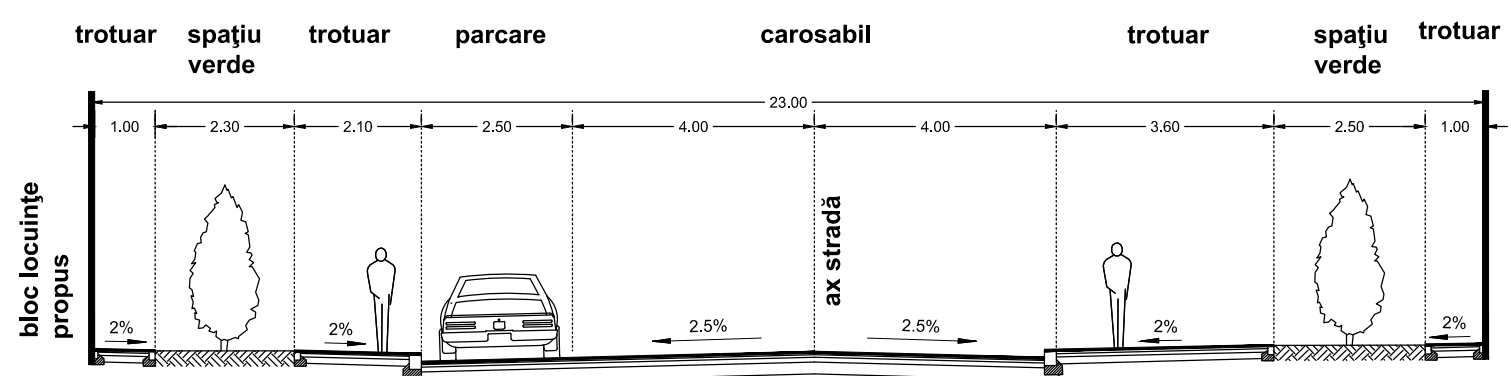
Secțiunea 2 Profil transversal
