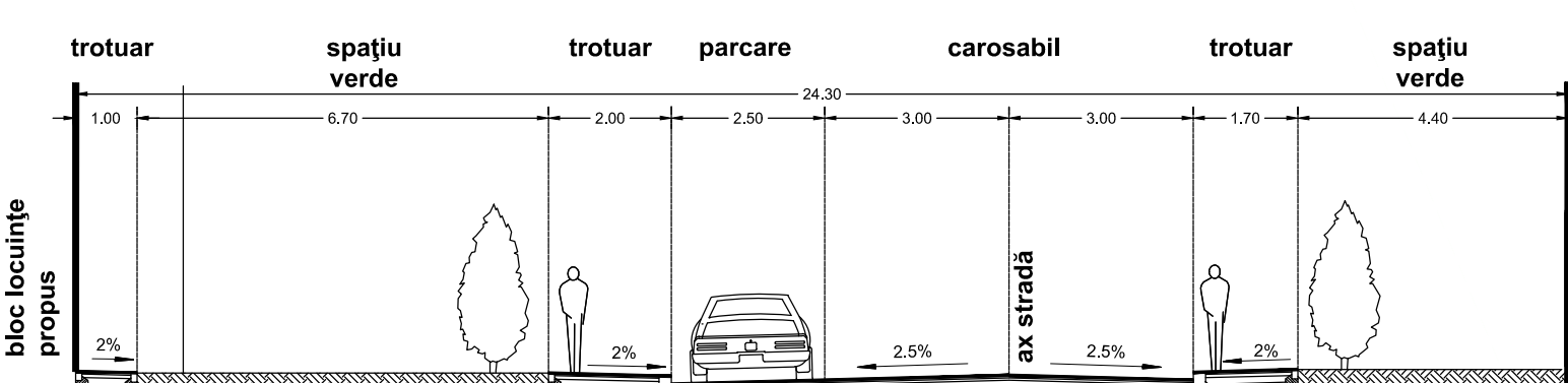
Secțiunea 5 Profil transversal
