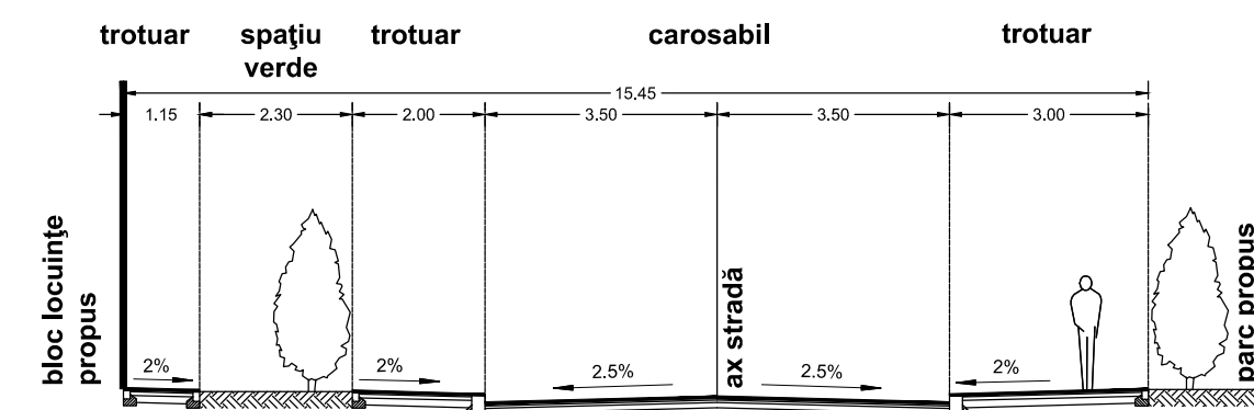
Secțiunea 7 Profil transversal
